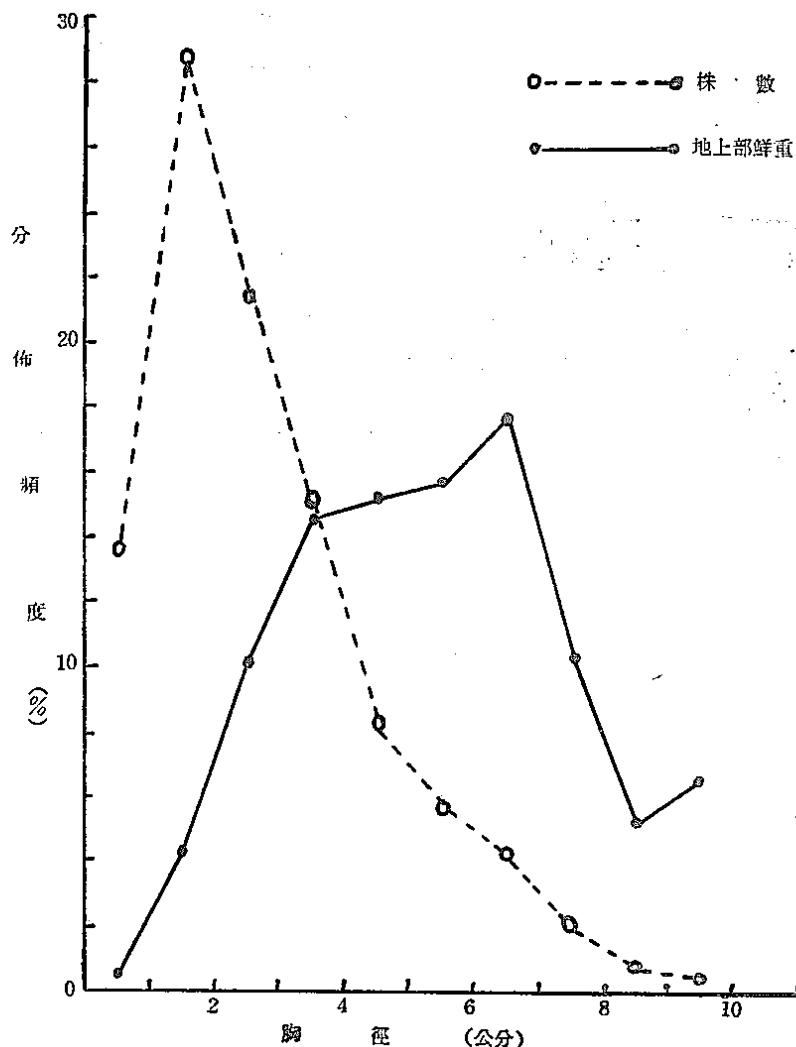
圖 1. 三民試區各胸徑級之株數與地上部乾重之分佈頻度。
