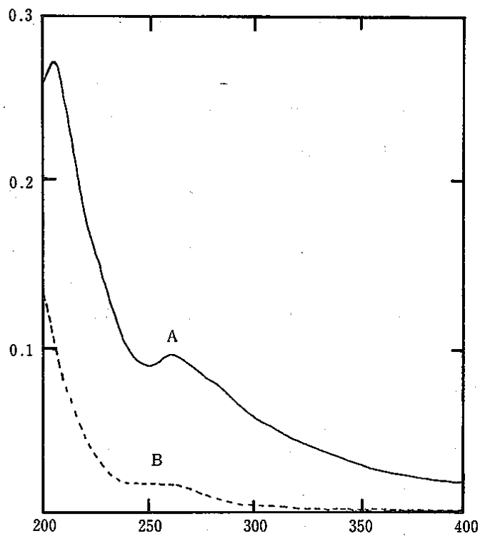
圖2 經照光後宣紙之水溶液與未經過照光宣紙水溶液之紫外線差異光譜圖。 ——，省產鑿宣；……，香港玉版單宣。
